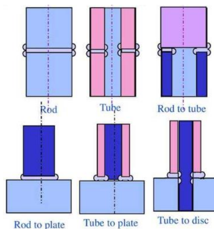
Gambar 5. Konfigurasi Sambungan Friction Rotary Welding
