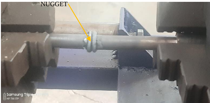
Gambar 8. Bentuk Material Uji Setelah Proses Pengelasan
