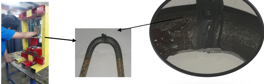
Gambar 11. Pengujian Bending
