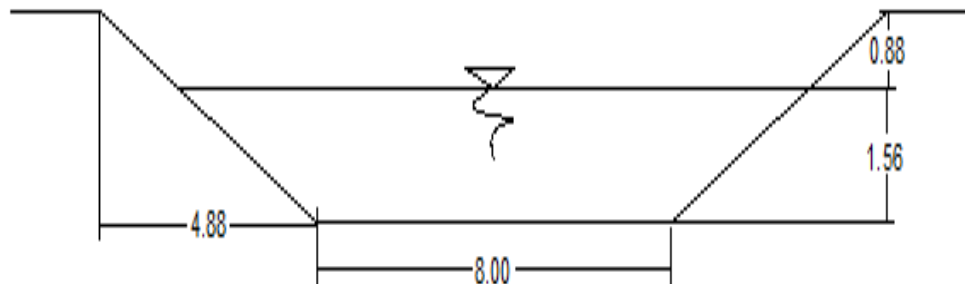
Gambar 7. Bentuk Dimensi Saluran Exiting (Efisien)
