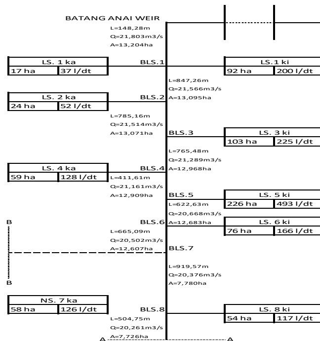
Gambar 3. Skema Jaringan
