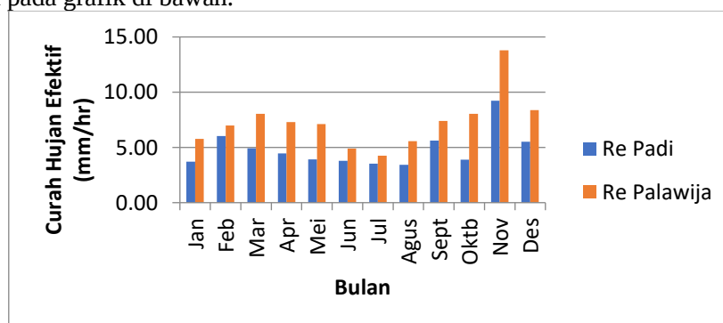
Gambar 1. Grafik Curah Hujan Efektif
